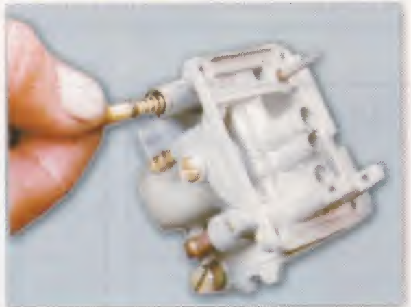
Colocación de la aguja para regulación de aire
